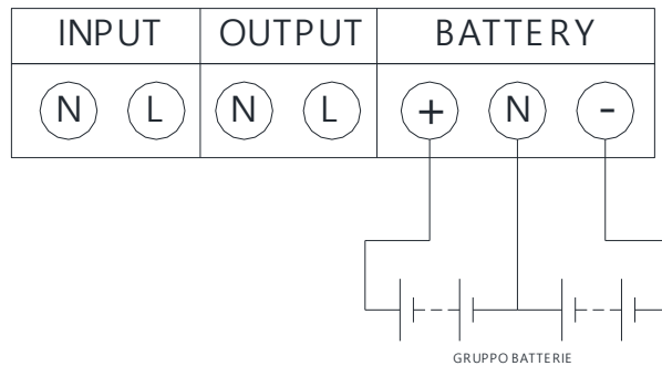
Fig.3 Connessioni morsettiera
