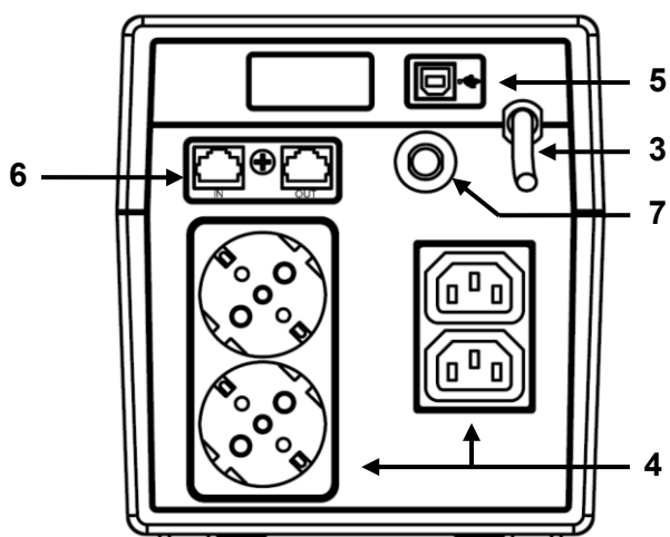
Vista posteriore UPS NemoLCD 160
