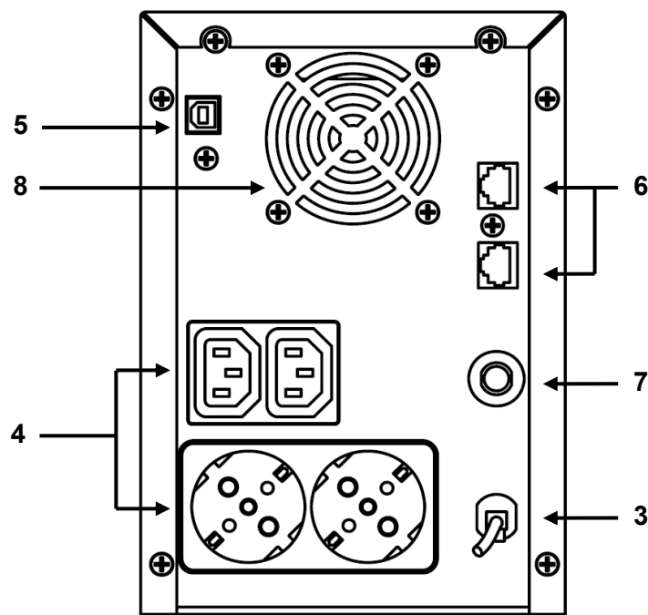
Vista posteriore UPS NemoLCD 400
