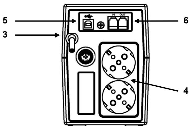
Vista posteriore UPS NemoLCD 65-80-120
