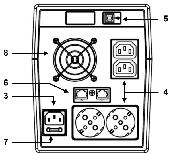
Vista posteriore UPS NemoLCD 200-300
