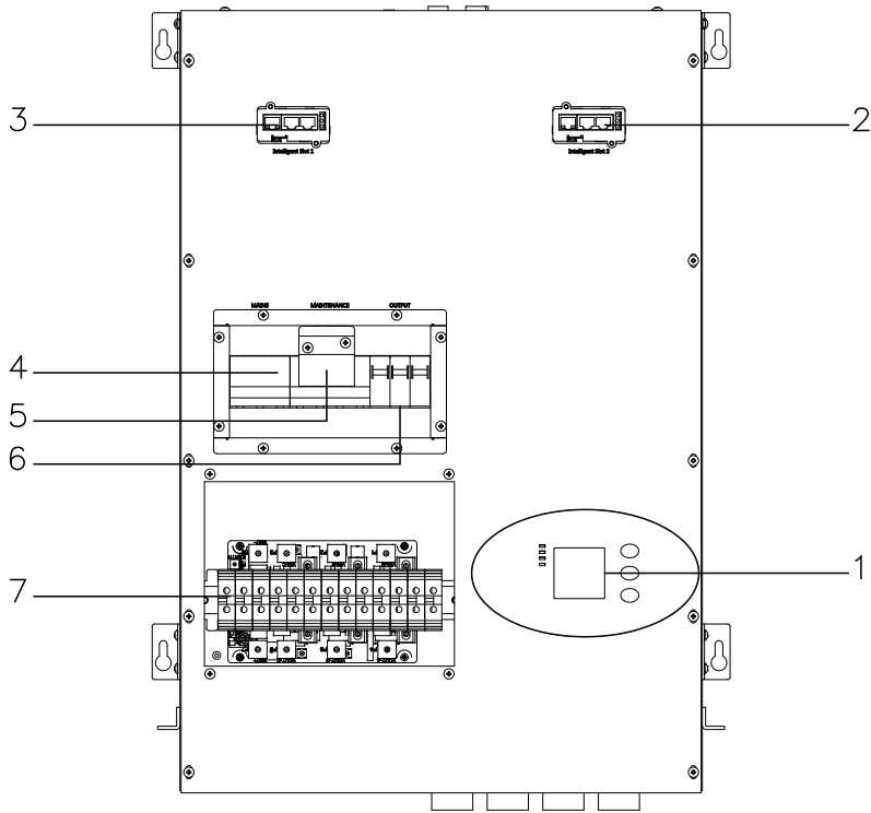
Vista Frontale con morsettiera
