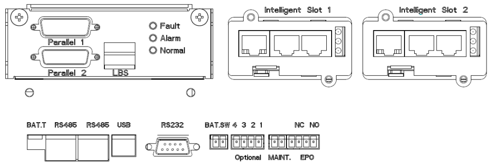
Vista superiore
