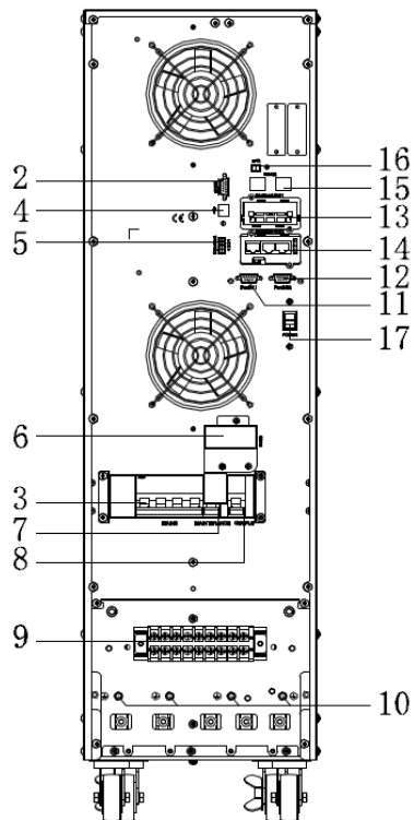
Vista Posteriore 10kVA (morsettiera senza coperchio)
