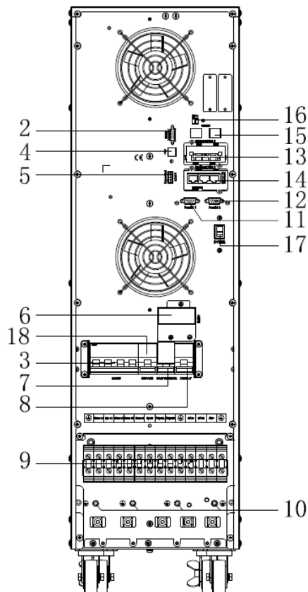
Vista Posteriore 15-20kVA
