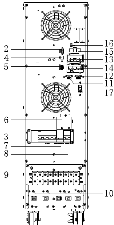
Vista Posteriore 15-20kVA (morsettiera senza coperchio)
